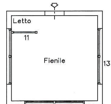
Pianta piano primo
