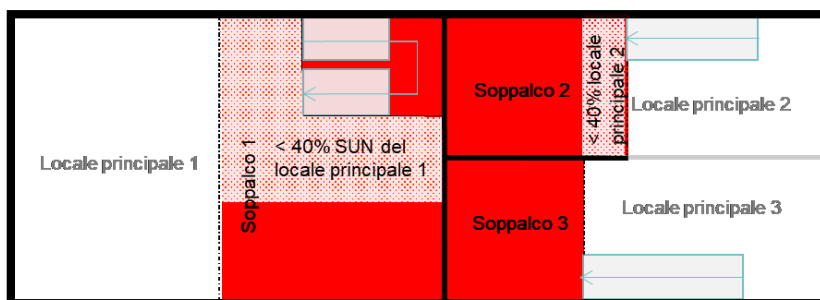
Figura 10 Il diagramma illustra un soppalco con una pendenza superiore al 30%. La distanza verticale tra il piano di calpestio e il piano di copertura è indicata come > 2,20 . La distanza orizzontale tra il muro di sostegno e il muro di chiusura è indicata come > 1,50 . La pendenza della copertura è indicata come p > 30\% . La zona sopraelevata è etichettata "Soppalco".
