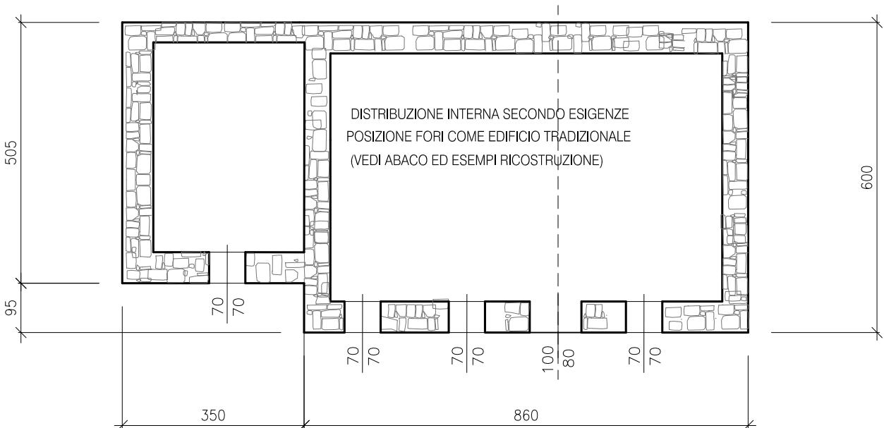
SCHEMA RECUPERO
